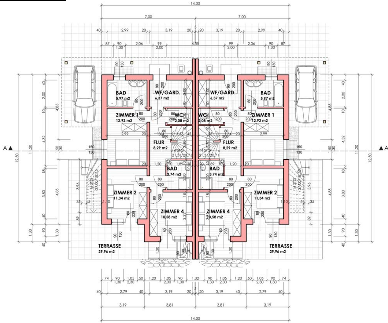
GRUNDRISS ERDGESCHOSS HAUS A
